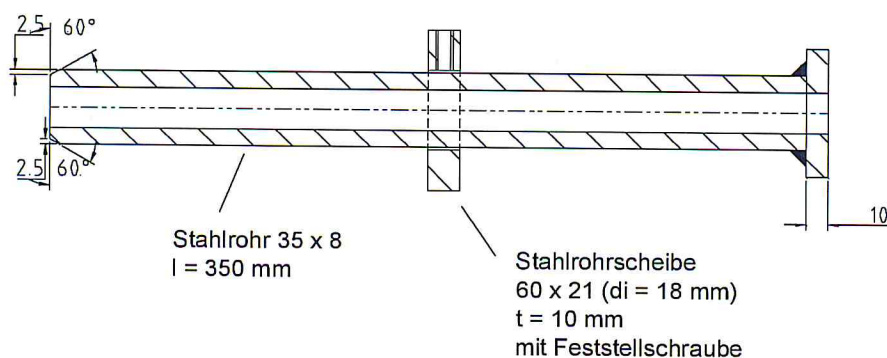
Bild 8: Setzwerkzeug
